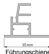
Führungsschiene
